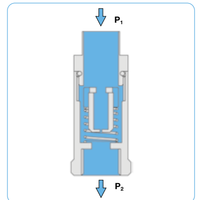
Schnittbild
